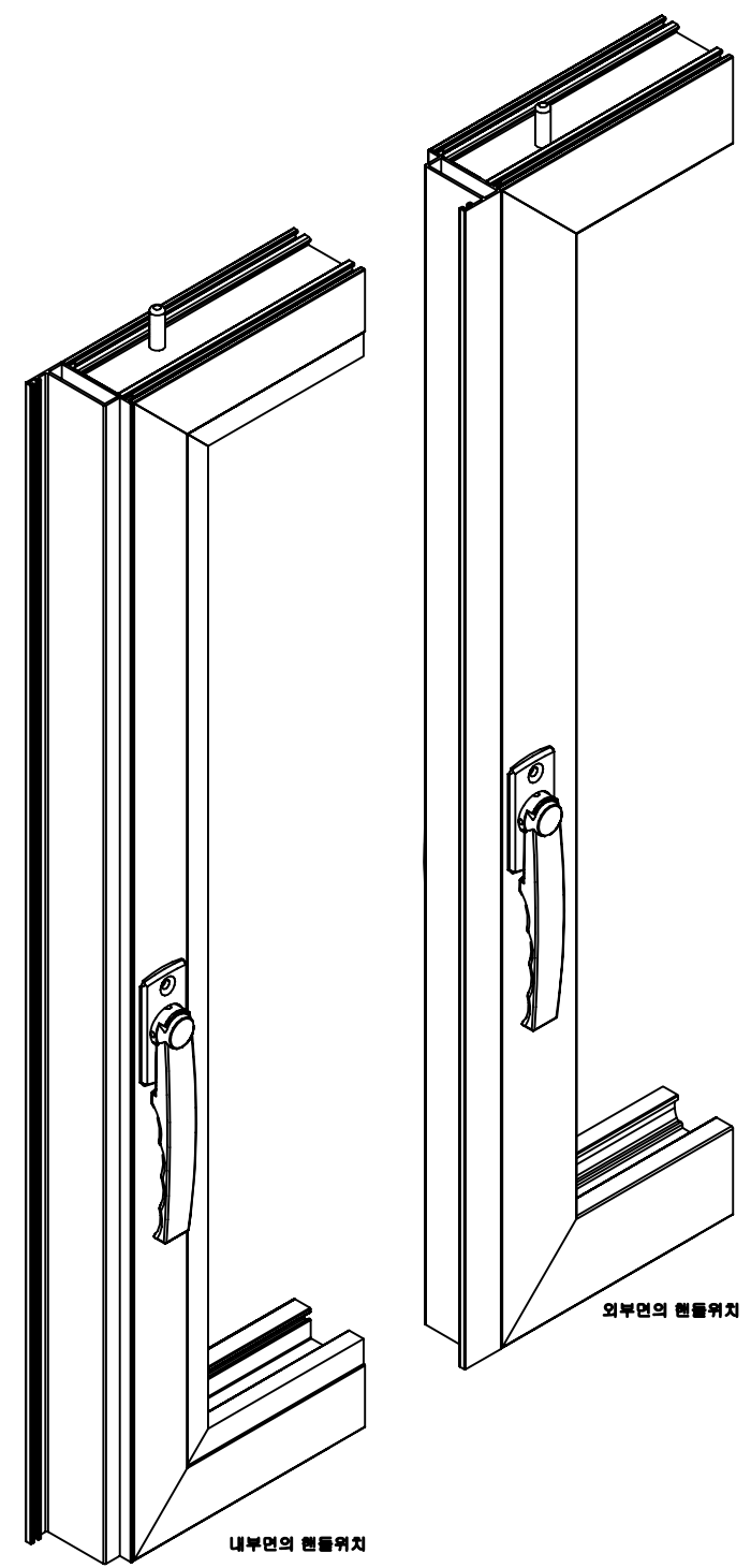
○ 닫힘 핸들 위치 SC | A1 : 1/2 ○ 열림 핸들 위치 SC | A1 : 1/2 ○ 닫힘 핸들 위치 SC | A3 : 1/4 ○ 열림 핸들 위치 SC | A3 : 1/4
