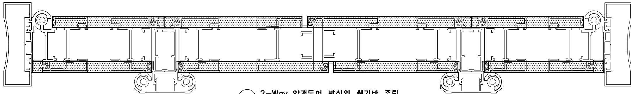
2-Way 양개도어 방식의 쉼기바 조립 SC | A1 : 1/1 SC | A3 : 1/2
