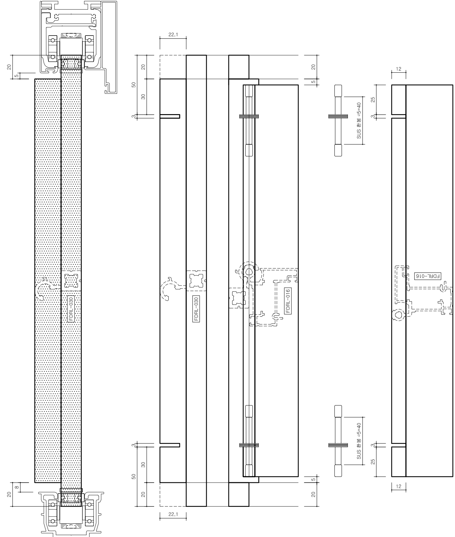
0 슬라이드 라인힌지 조립 상세도 SC | A1 : 1/1 SC | A3 : 1/2
