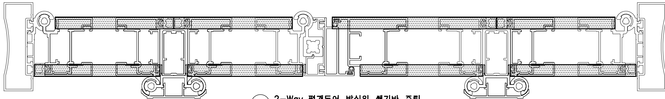
2-Way 팬개도어 방식의 쉼기바 조립 SC | A1 : 1/1 SC | A3 : 1/2
